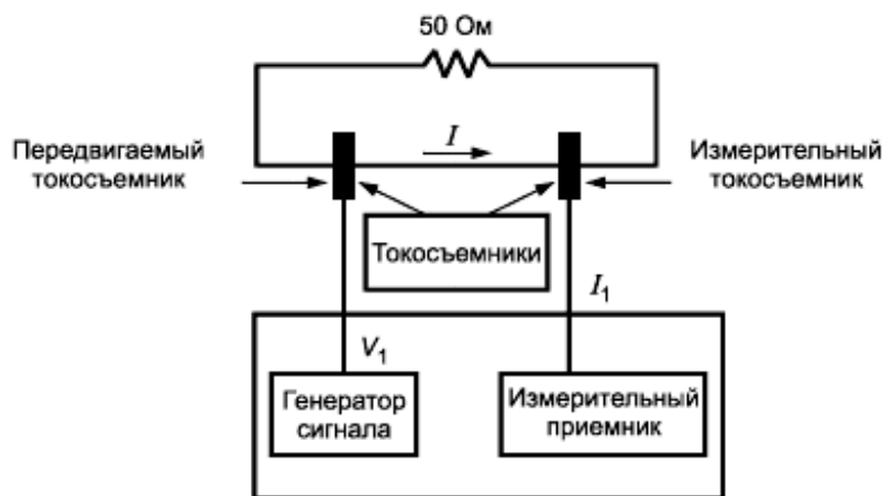
Рисунок А.5 - Схема калибровки
