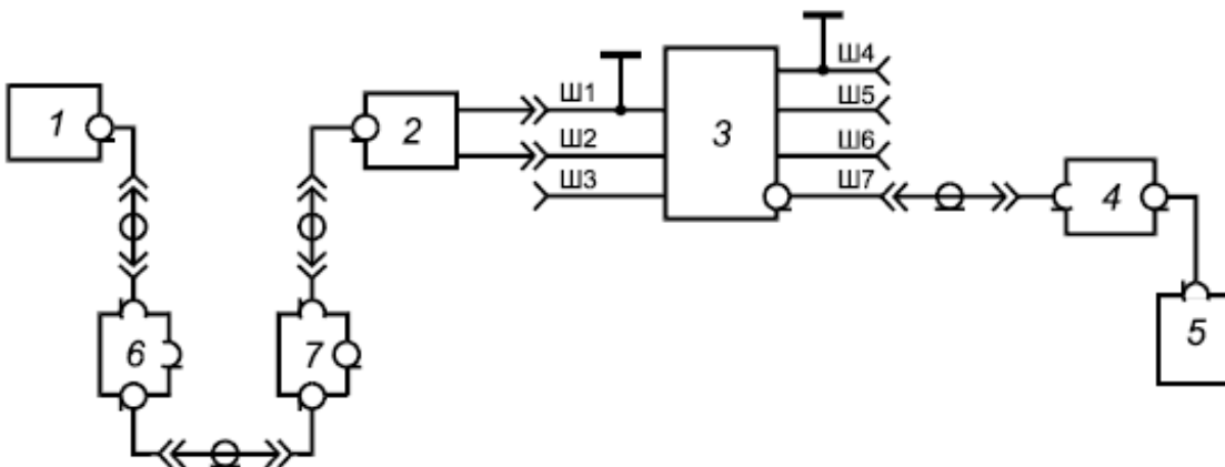
б) Схема измерения напряжения U_1
